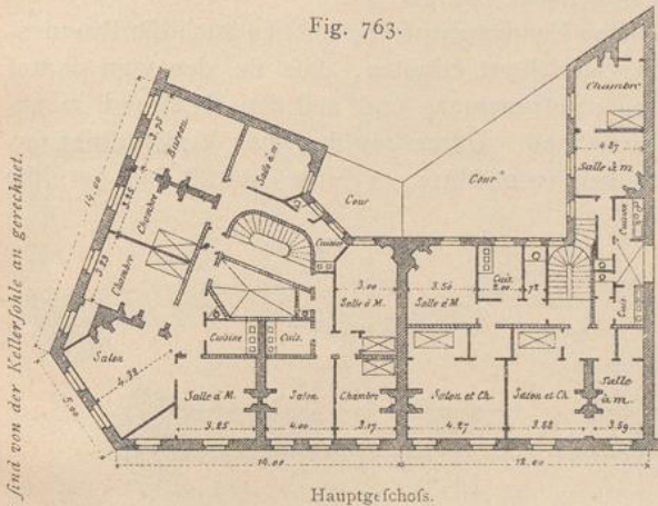
Hauptgeschoss.
