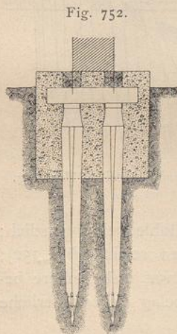
Vom Leichenschauhaus zu Paris 260 ). — 1/50 w. Gr.
