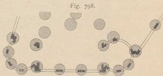
Von den Magasins du Printemps zu Paris. Teil des Fundamentplanes 283) . — 1/500 w. Gr.
