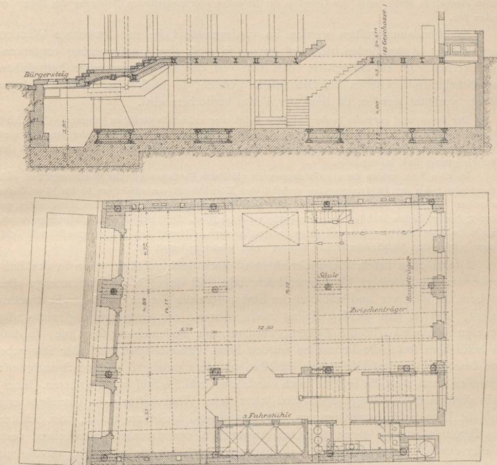
Gründung eines Gefchäftshaufes in der Pine-Street zu New-York 232) . — 1/150 w. Gr.
