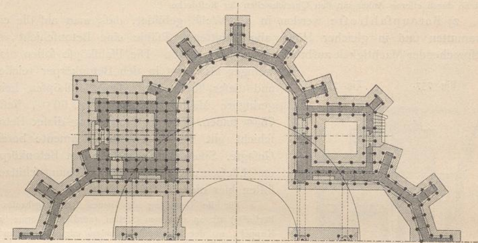
Von der neuen protestantischen Kirche zu Badenweiler 263) .
