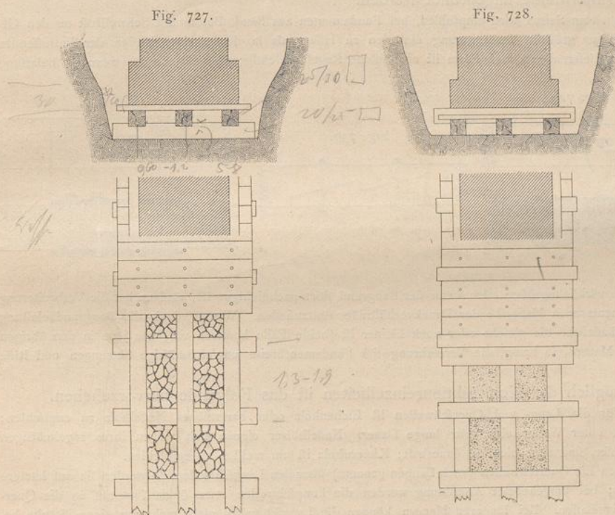
Schwellroste. — \frac{1}{100} W. Gr.
