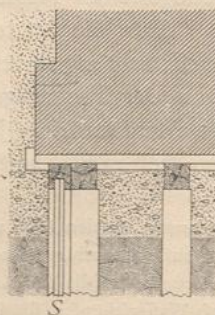
Anordnung von Spundwänden bei Pfahlrosten. — 1/100 w. Gr.
