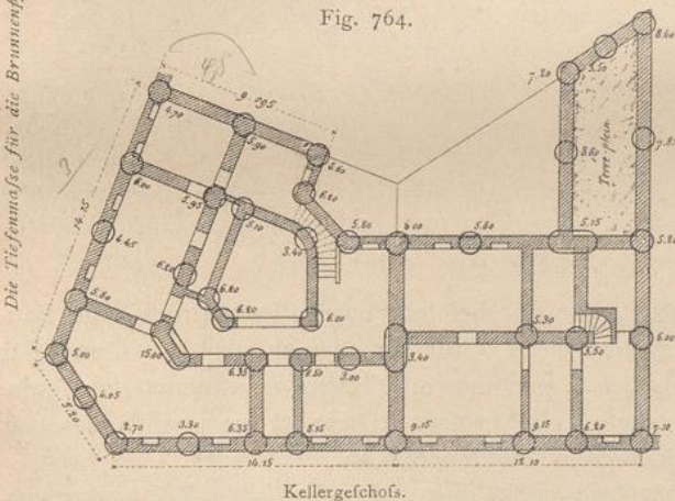
Kellergeschoß.
