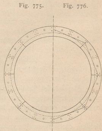
Brunnenkranz. — \frac{1}{50} w. Gr.
