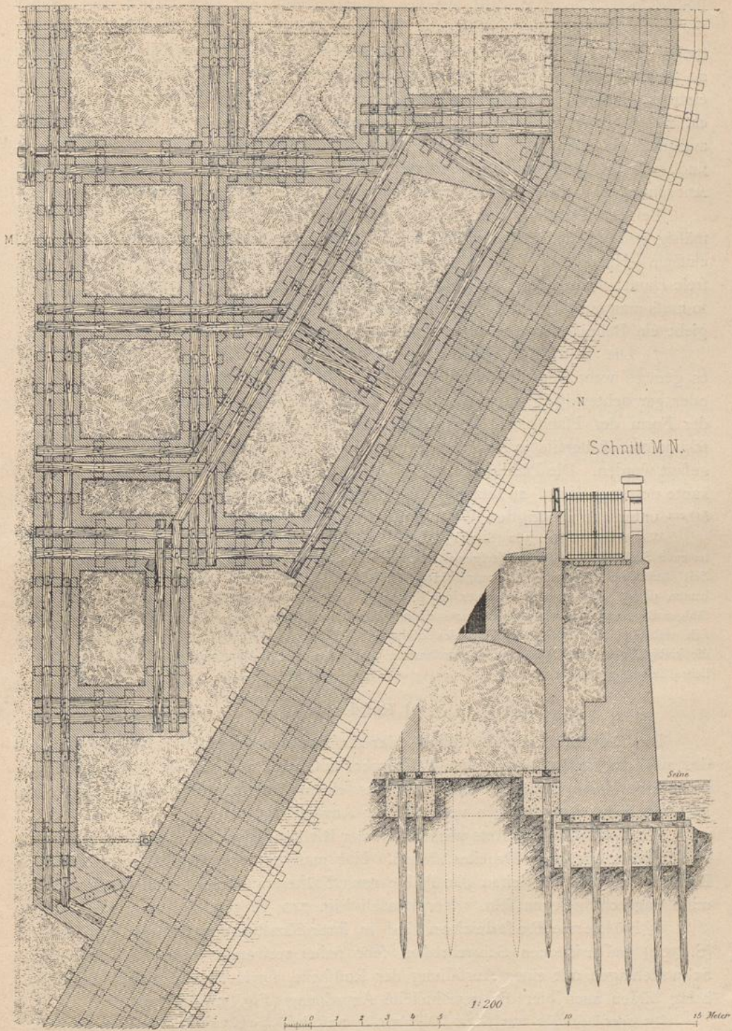
Fundamentplan des Leichenschauhauses zu Paris. — Südliche Hälfte 250) .
