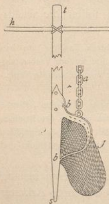
Sackbohrer.
