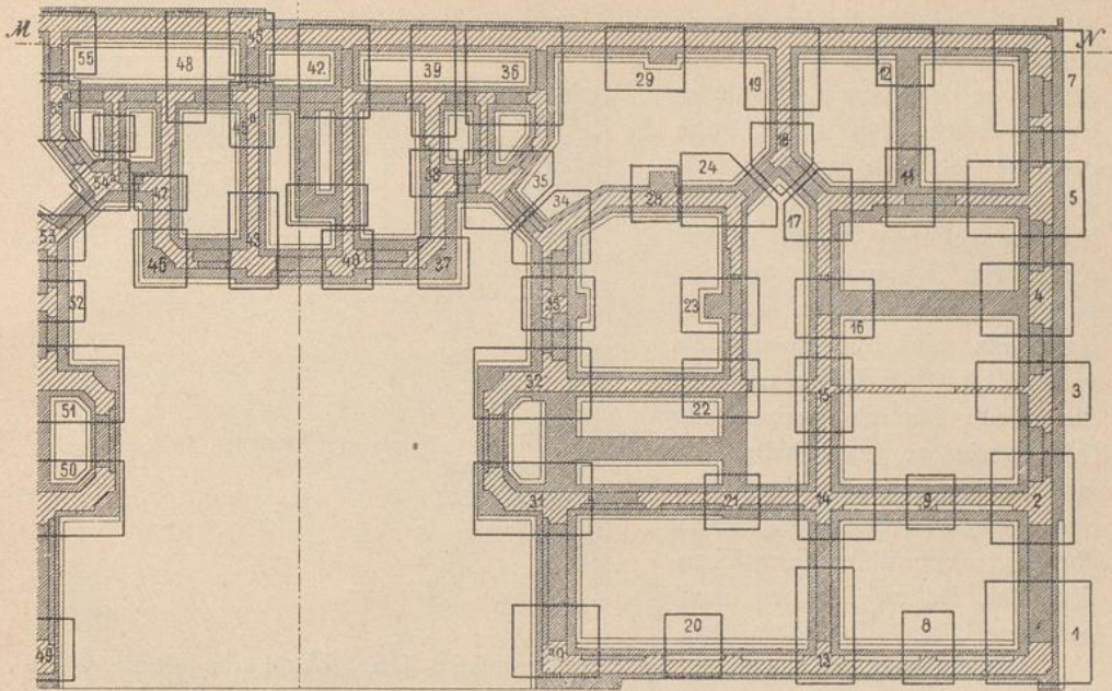
Grundriss des Erdgeschosses und Fundamentplan. — 1/200 w. Gr.
