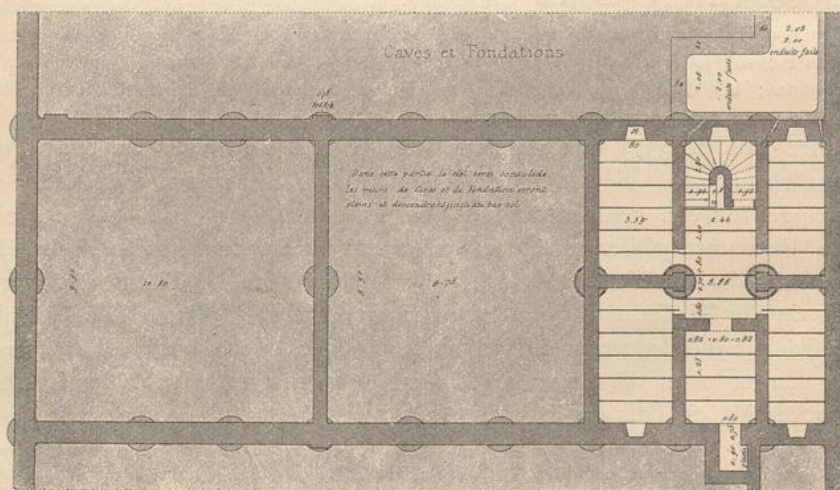
Fundamentplan.
