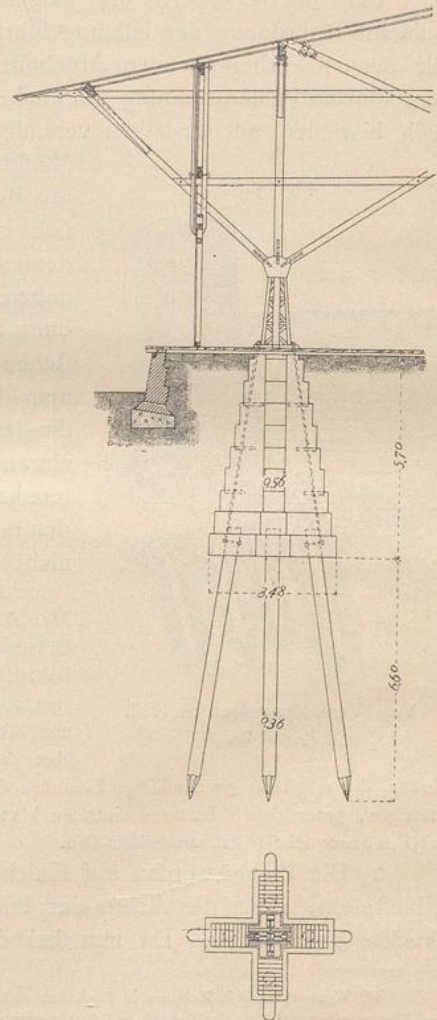
Vom Quaischuppen am Grasbrookhafen zu Hamburg. — 1/200 w. Gr.
