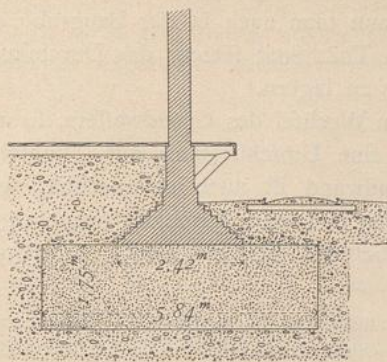
Vom Güterschuppen auf dem Bahnhofe zu Emden 240) .
