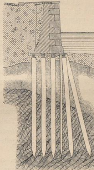
Reefendamm-Quaimauer zu Hamburg. — 1/200 w. Gr.
