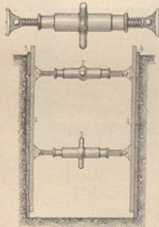
Abspriesswinde von Karl Birmel zu Freiburg i. B.
