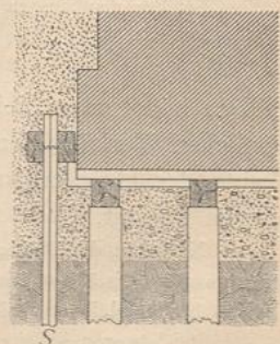
Anordnung von Spundwänden bei Pfahlrosten. — 1/100 w. Gr.
