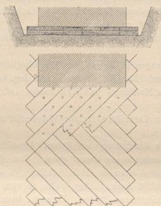
Doppelte Bohlenroste.
