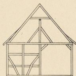
Abb. 8. Querschnitt.
