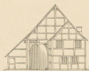
Abb. 10. Haus Nr. 14 (Pieper) in Heyen. Südseite.
