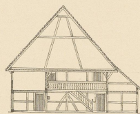
Abb. 3. Sonnenberg. Querschnitt AB.
