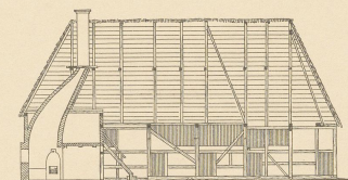
Abb. 7. Boimsdorf. Längenschnitt A B.
