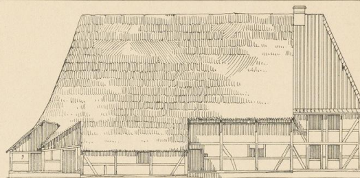
Abb. 2. Haus Müller in Velpke. Längenschnitt.
