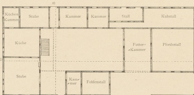
Abb. 5. Sonnenberg. Grundriss.
