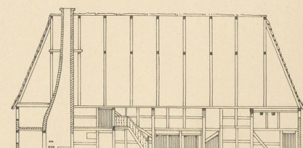
Abb. 23. Haus Wolter in Lehre. Längenschnitt.
