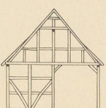
Abb. 10. Giebelansicht.
