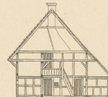
Abb. 11. Wahrstedt. Schnitt AB.
