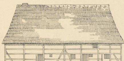
Abb. 22. Haus Wolter in Lehre. Längenschnitt.
