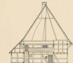
Abb. 4. Velpke. Querschnitt.
