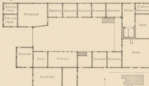
Abb. 3. Haus Müller in Velpke von 1675. Grundriss.
