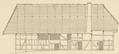
Abb. 3. Haus Warnecke in Glentorf (1703). Längenschnitt A B.
