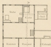
Abb. 2. Bremke. Grundriss.
