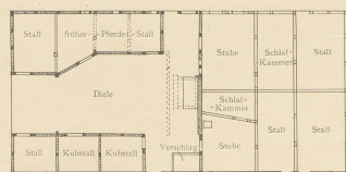
Abb. 13. Haus Nr. 12 in Neubrück (1660).
