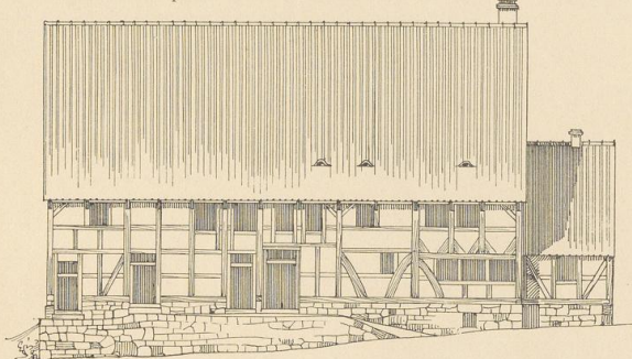
Abb. 17. Haus Schilling in Dankelsheim. Längenschnitt.
