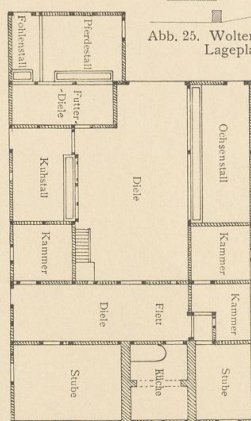
Abb. 24. Haus Wolter in Lehre.
