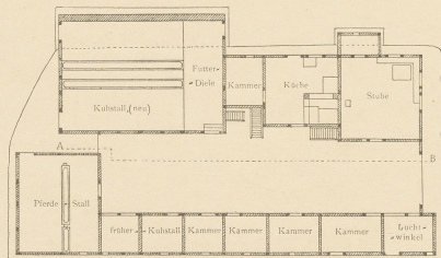
Abb. 5. Glentorf. Grundriss.
