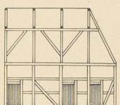
Abb. 9. Längenschnitt.
