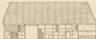
Abb. 4. Sonnenberg. Längenschnitt CD.
