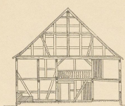
Abb. 1. Haus in Bremke (um 1700). Querschnitt A B
