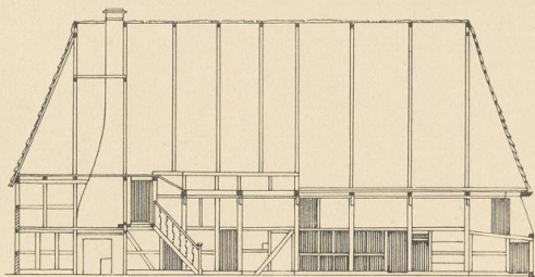
Abb. 1. Haus Müller in Velpke. Längenschnitt.
