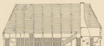
Abb. 15. Bergfeld. Längenschnitt AB.
