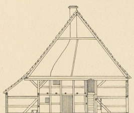
Abb. 21. Wolter in Lehre. Querschnitt.
