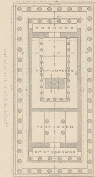
2. Grundriss des Parthenon. (Nach Dörpfeld.)
