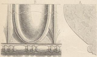
10. Ionisches Kymation.
