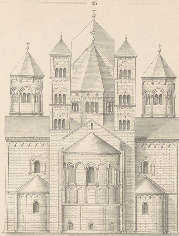
5. Abteikirche zu Laach. Oestlicher Aufriss. 1100-1150
