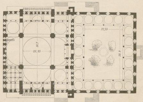
4. Mahmud's II, Moschee. Grundriss. (Constantinopel.)
