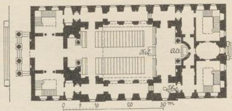
Abbildg. 773 u. 74. Schloßkirche in Kopenhagen. Erbaut durch C. F. Hansen 1826.
