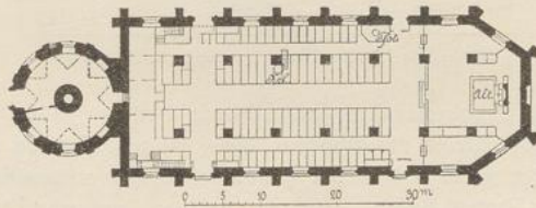
Abbildg. 763. Dreifaltigkeits-Kirche in Kopenhagen. Erbaut 1637—56.
