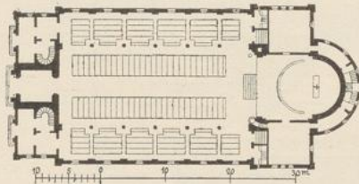
Abbildg. 776. St. Pauls-Kirche in Kopenhagen. Erbaut durch Gmudhmann 1872—77.
