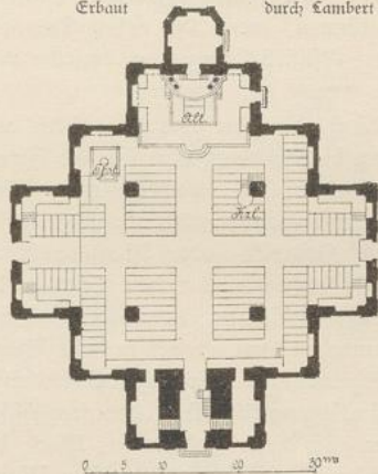
Abbildg. 765 u. 66. Erlöser-Kirche (Vor freisers-K.) in Kopenhagen. Erbaut durch Lambert v. Haven 1682—94. (Thurmspitze 1749/50.)
