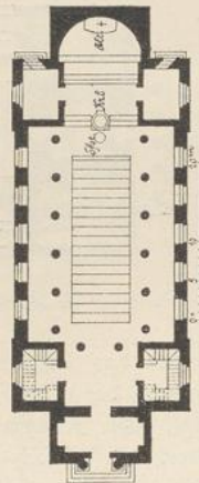
Abbildg. 770. Kirche in Hörsholm. Erb. d. C. F. Hansen 1820-23.
