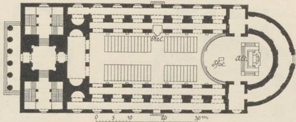
Abbildg. 77 ( u. 72. Frauen-Kirche in Kopenhagen. Erbaut durch Chr. Fr. Hansen 1811—29.
