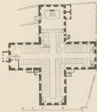
Abbildg. 759. Holmens-Kirche in Kopenhagen. Erbaut 1619—41.
