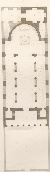
Grundriß der Kirche von S. Erze in Gumbinnen Plan de la Paroisse de S. Erze de Gumbinnen Piano della Chiesa di S. Erze in Gumbinnen
