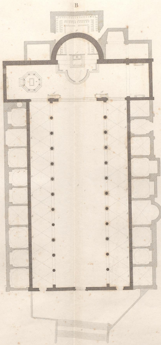
Grundriß der Kirche von S. Maria in Arcove Plan de l'église de S. Marie à Arcove Piano della Chiesa della Santa in Arcove
