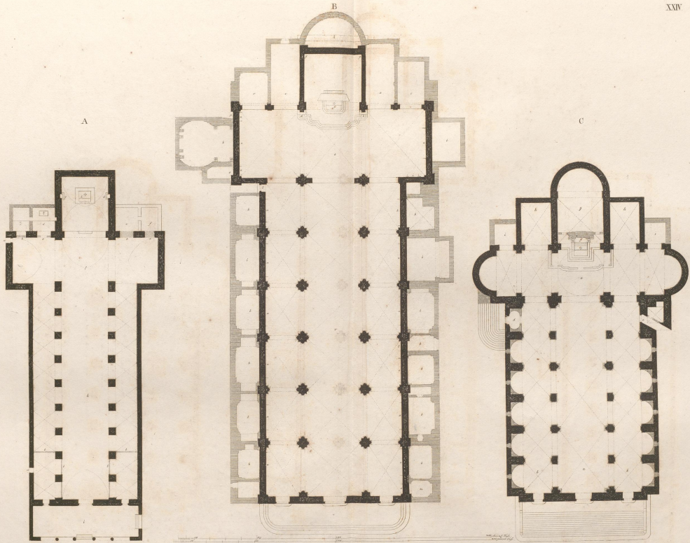
Grandi del Sordani con l'incisa alla Fontana Plan de l'eglise de l'Anquet aux trois Fontaines Plan de la Chiesa de S. Vincenzo alle tre Fontane
