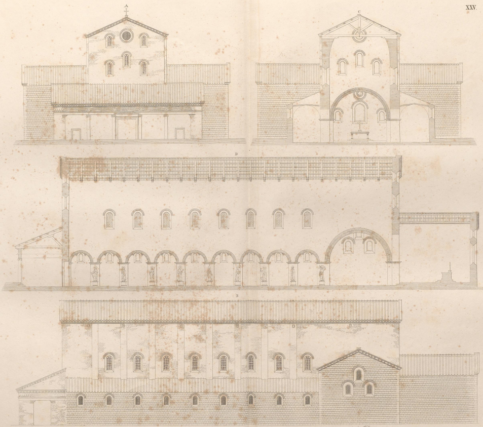
Ansichte und Querschnitt von der Kirche St. Vincent alle tre Fontane. Facade et Coupe de l'Eglise de St. Vincent aux trois Fontaines. Faciata e spaccato della Chiesa di S. Vincenzo alle tre Fontane.
