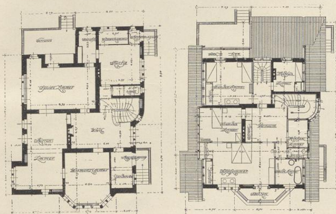
4. Grundriß des Erd- und des I. Obergeschosses eines Hauses in Darmstadt. Von Alfred Messel. (Muthesius, Landhaus und Garten.)
