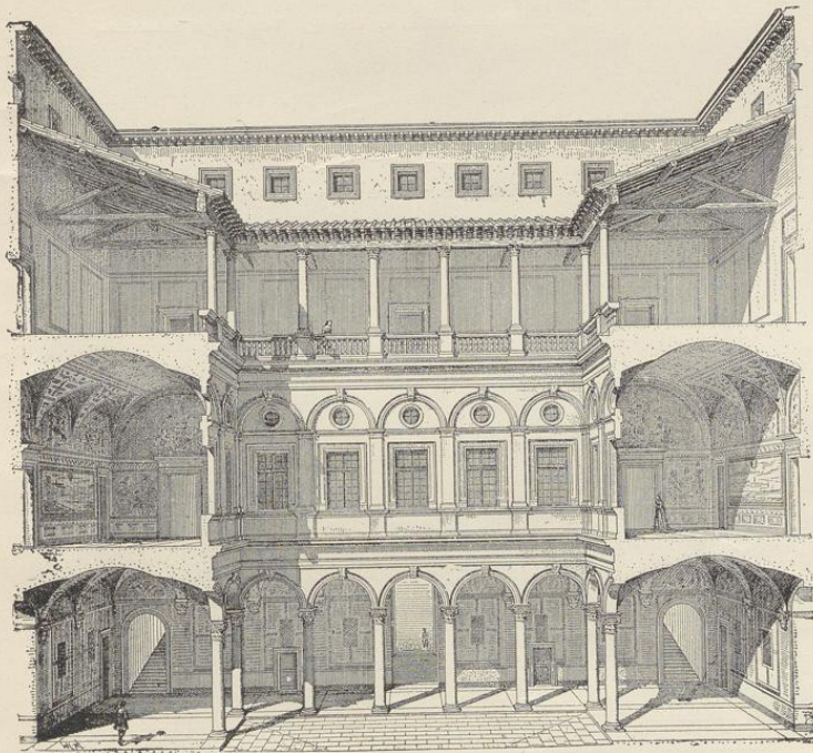
5. Schnitt durch den Hof des Palazzo Strozzi in Florenz.
