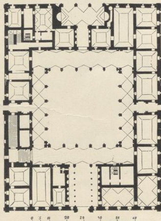
3. Grundriß des Palastes Farnese in Rom.
