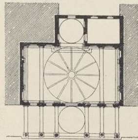
4. Grundriß der Cappella de' Pazzi zu Florenz.
