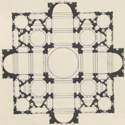
2. Bramantes Plan zur Peterskirche in Rom.
