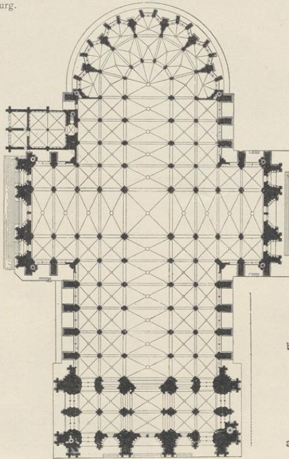
3. Grundriß des Kölner Domes.
