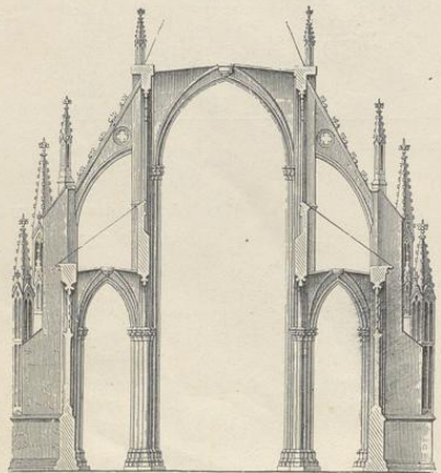
8. Querschnitt des Domes zu Halberstadt.
