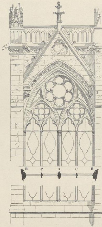
4. Fenster mit Wimperg von der Ste. Chapelle zu Paris. A. Alter Pfosten. BB. Wandpfosten. CC. Junge Pfosten.
