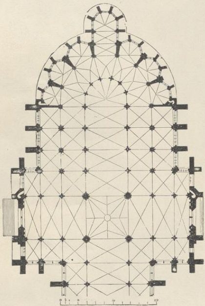
2. Grundriß der Kathedrale zu Amiens.
