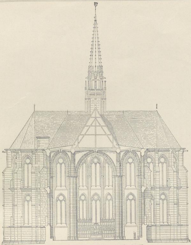
1. Querschnitt der Elisabethkirche zu Marburg. (Nach Moller.)
