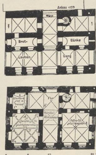
6. Rathaus zu Marienburg. Erdgeschoß und Obergeschoß. (Nach B. Schmidt. »Die Denkmalpflege«, Jahrg. 1902.)
