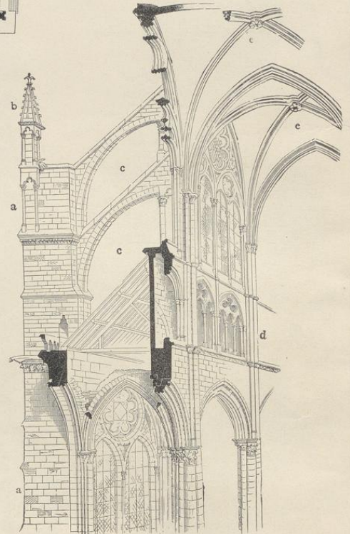
7. Gewölbesystem der Kathedrale zu Amiens. a. Strebepfeiler. b. Fiale. cc. Strebobogen. d. Triforium. ee. Kreuzgewölbe.
