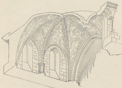
3. Sechsteiliges Rippengewölbe. (Dehio u. v. Bezold.)
