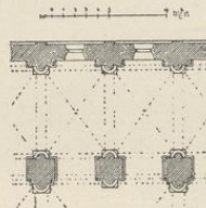
4. Gewölbesysteme der Dome zu Mainz (a) und Speyer (b).
