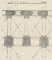
4. Gewölbesysteme der Dome zu Mainz (a) und Speyer (b).
