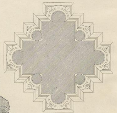
17. Grundriß eines gegliederten Pfeilers. (Dom zu Naumburg.)
