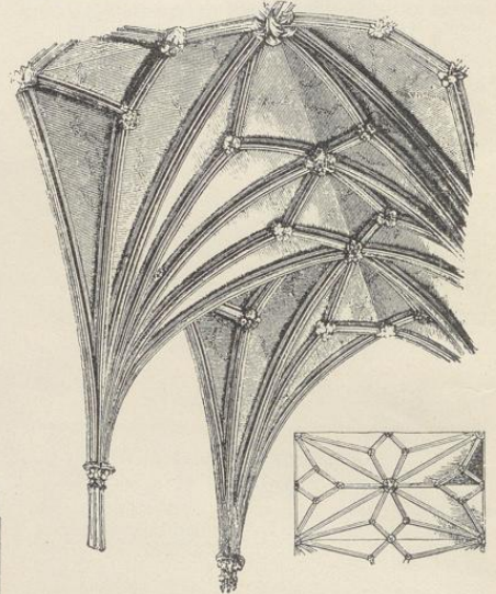
5. Sterngewölbe. (Nach Parkers Glossary.)
