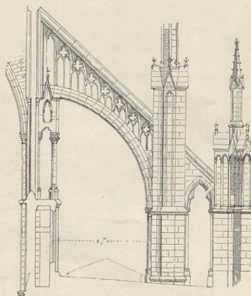
6. Strebeystem am Chor der Kathedrale zu Amiens.
