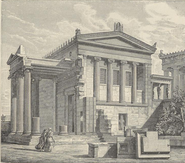
6. Nordwestansicht des Erechtheions. (Nach Niemann.)
