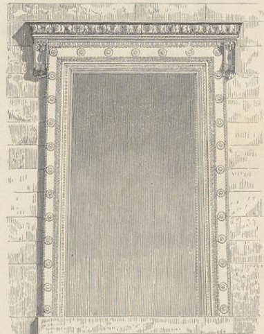
5. Fenster und Türe vom Erechtheion.
