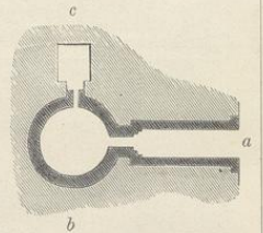
3. Schatzhaus des Atreus.
