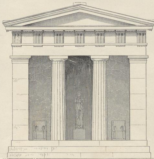
8. Der ältere Tempel der Nemesis zu Rhamnus.
