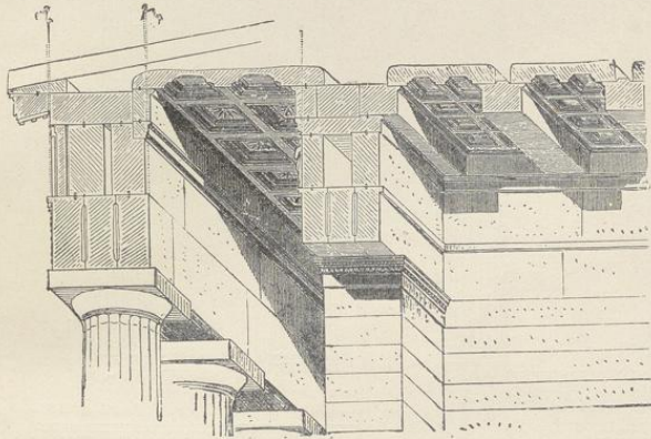
4. Deckenbildung des dorischen Tempels. (Nach Durm.)
