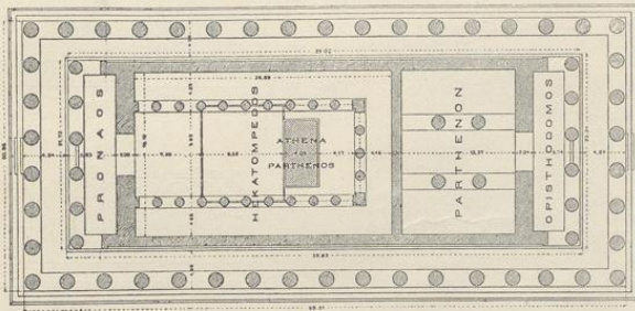
12. Grundriß des Parthenons. (Nach Dörpfeld.)
