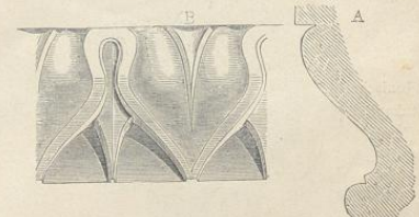
11. Herzblatt (Lesbisches Kymation).
