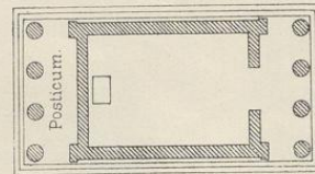
10. Amphiprostylos.
