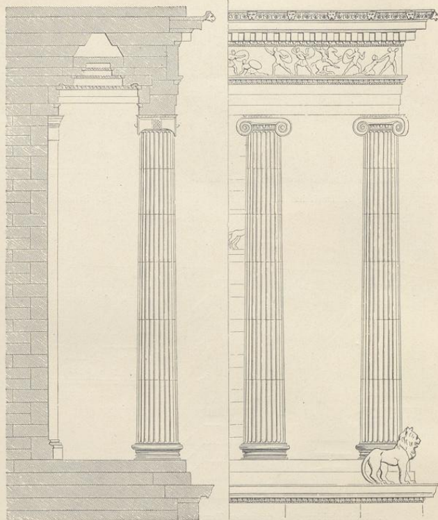
2. Schnitt und Ansicht von der Säulenhalle zu Halikarnass.
