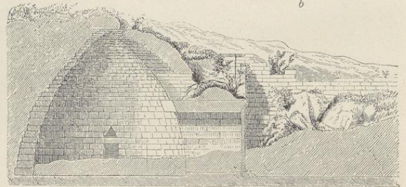
4. Sogen. Schatzhaus des Atreus. Grabtempel bei Mykenae.
