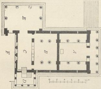
4. Grundriß des Erechtheions auf der Akropolis zu Athen (ca. 410 v. Chr.)
