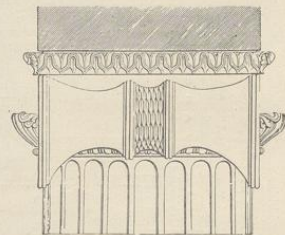
4. Seitenansicht des jonischen Kapitäl.
