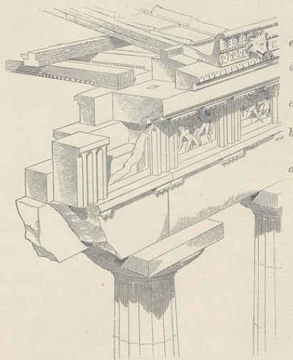
5. Dorische Deckenbildung. a. Architrav (Tragbalken), b. Tropfen, c. Triglyphenfries, d. Kranzgesims (Geison), e. Rinnleiste (Sima).
