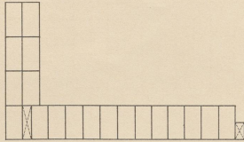
Blockverband bei Anwendung von Kopfstücken.
