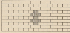
Blockverband bei Anwendung von Kopfstücken.
