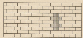
Blockverband bei Anwendung von Dreiviertelsteinen.
