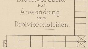
Diese Verbände für rechtwinklige Pfeiler gelten zugleich für die Mauerbögen.
