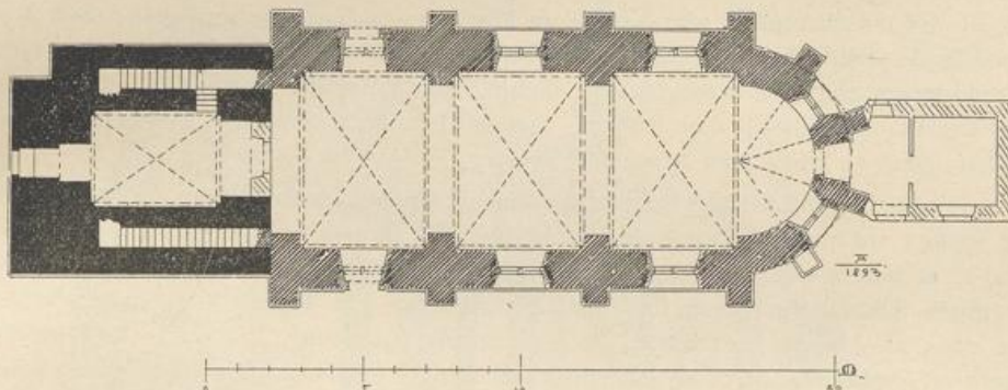
Fig. 17. Marienhagen. Grundriss der evangelischen Pfarrkirche.
