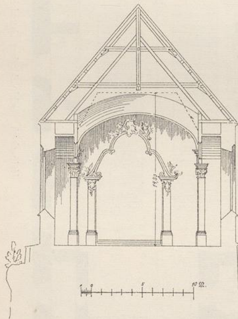
Haigerloch, Schlosskirche: Querschnitt.
