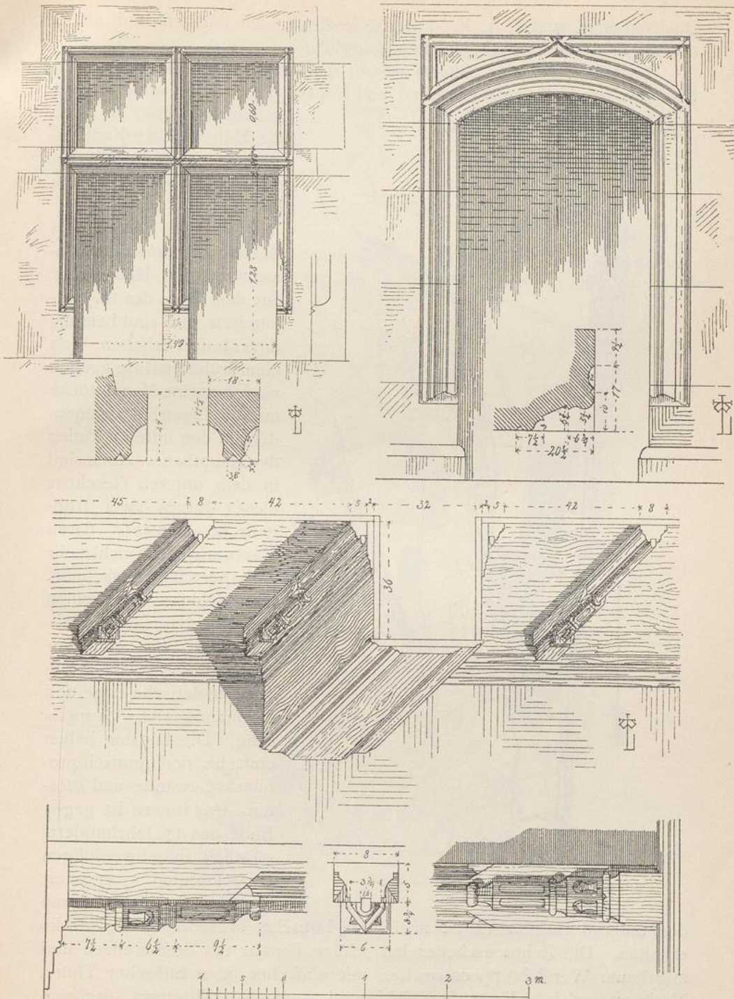
Haigerloch. Schloss: Fenster, Thüre und Balkendecke. Kunstdenkmale in Hohenzollern.
