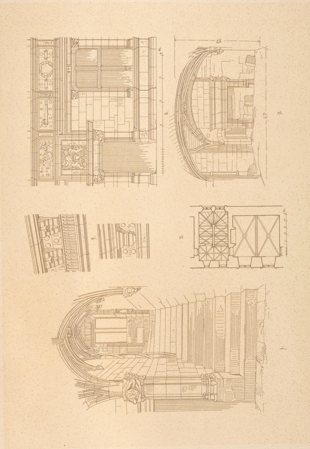
SCHLOSS. 1. TREPPENHAUS. 2. ZIMMER IM ERDGESCHOSS. 3. GRUNDRISS ZU 1. UND 2. 4. HAUPTGESIMSE. 5. ÄUSSERES ERDGESCHOSS.
