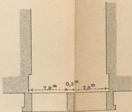
Fig. 287. Grundriss.
