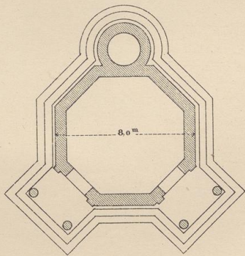
Fig. 284. Grundriss.
