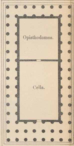
Pseudodipteros.
