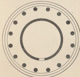
Monopteros. (Centralperipteros.)
