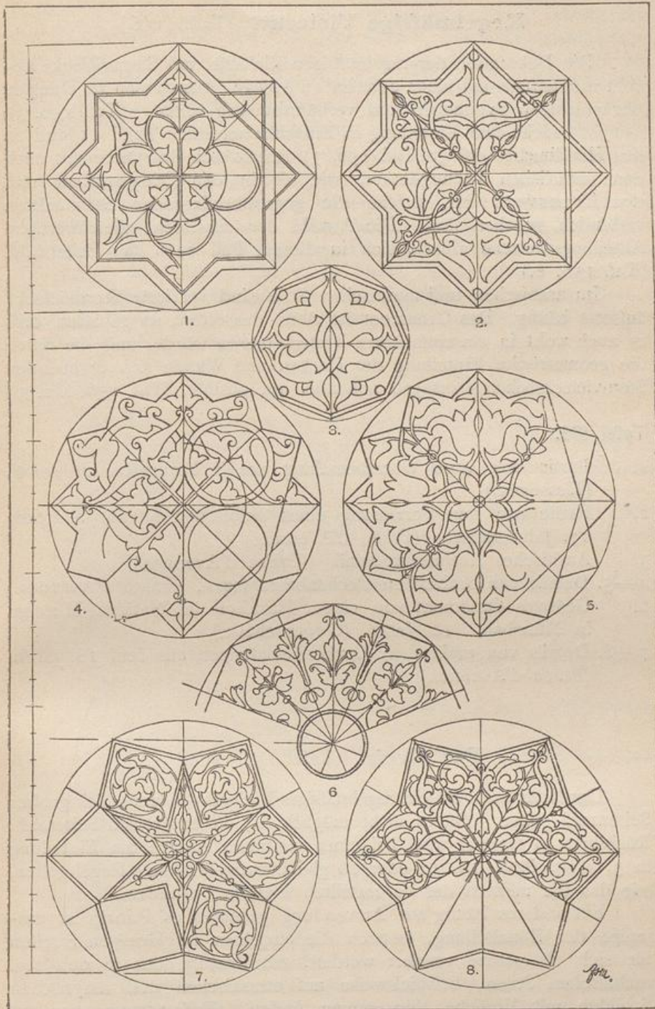
Regelmäßige Vielecke.
