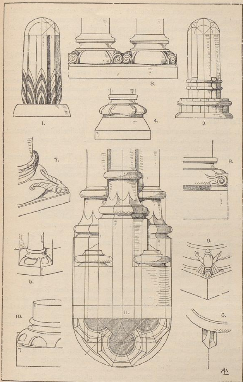
Säulenfüße.
