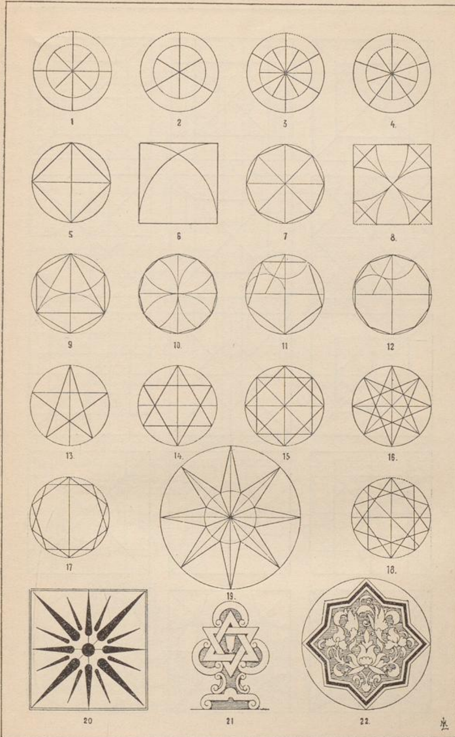
Vielstrahl, Vielecke und Sternvierecke.
