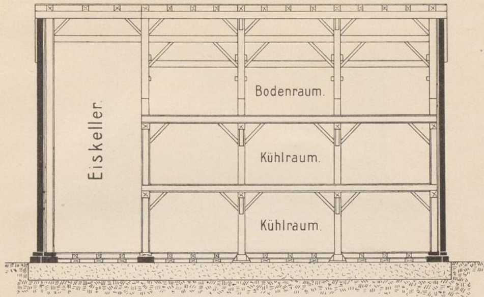
Schnitt C—D.
