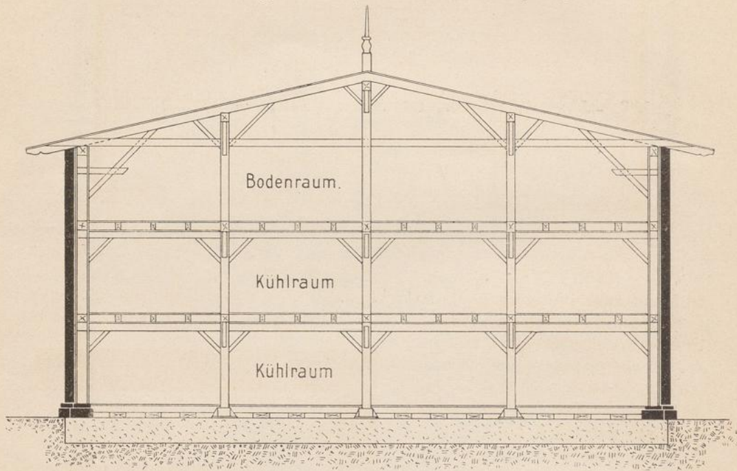
Schnitt A—B.
