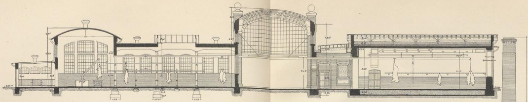
• SCHNITT A-B •
