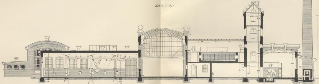
• SCHNITT C-D •
