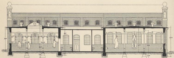
• SCHNITT E-F •
