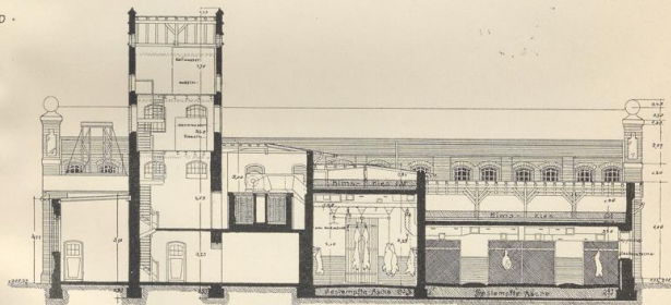
• SCHNITT G-H •
