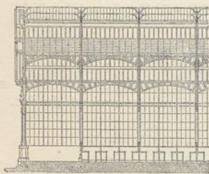
Fig. 276. Längenschnitt 194) .
