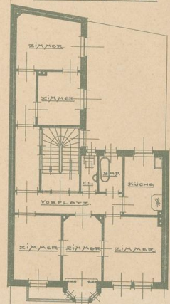
I. OBERGESCHOSS.
