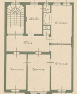
Erstgeschoss
