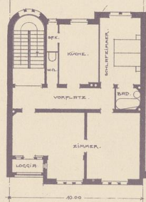
WOHNUNGSGESCHOSS.
