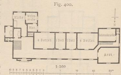
Kranken-Pflegehaus zu Wilster. Erdgeschoss 1755). 1869 u. 1879.
