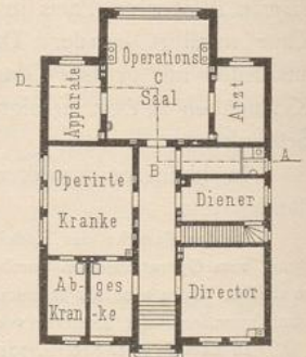
Erdgeschoß.
