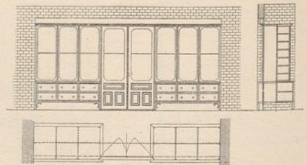
Instrumentenschrank im neuen allgemeinen Krankenhaus zu Hamburg-Eppendorf 1563) .
