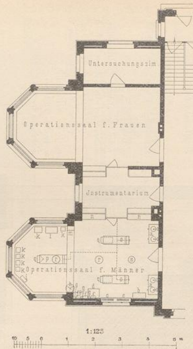
Großer Operationsaal im neuen allgemeinen Krankenhaus zu Hamburg-Eppendorf 1563) .
