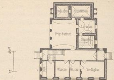
Badehaus im neuen städtischen Krankenhaus zu Nürnberg 1518) .
