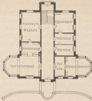
Operationsgebäude im neuen allgemeinen Krankenhaus zu Hamburg-Eppendorf (1866), Arch.: Zimmermann & Ruppel.
