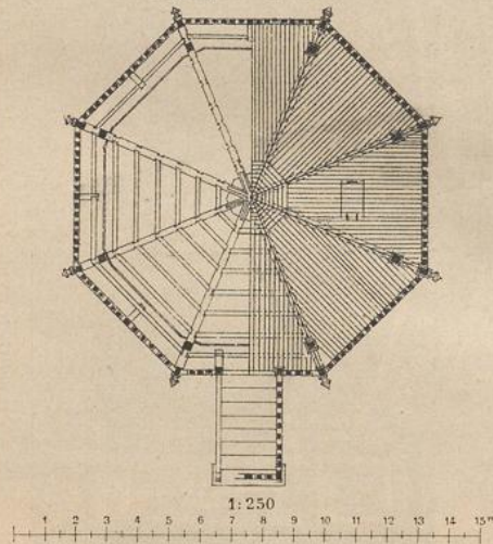
Fig. 460. Grundriß.
