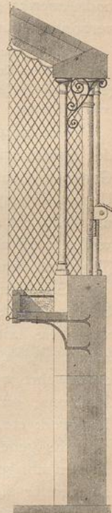
Schnitt durch die Galerie-Wand 392) . 1/25 n.-Gr.
