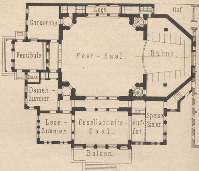
Bohnstedt's Entwurf zu einem Gesellschafts-Local für den Künstlerverein »Malkasten« in Düsseldorf 342) .
