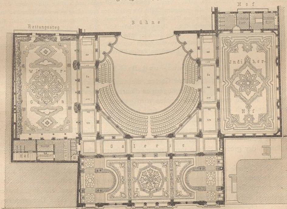
Fig. 143. Hauptgefchofs.
