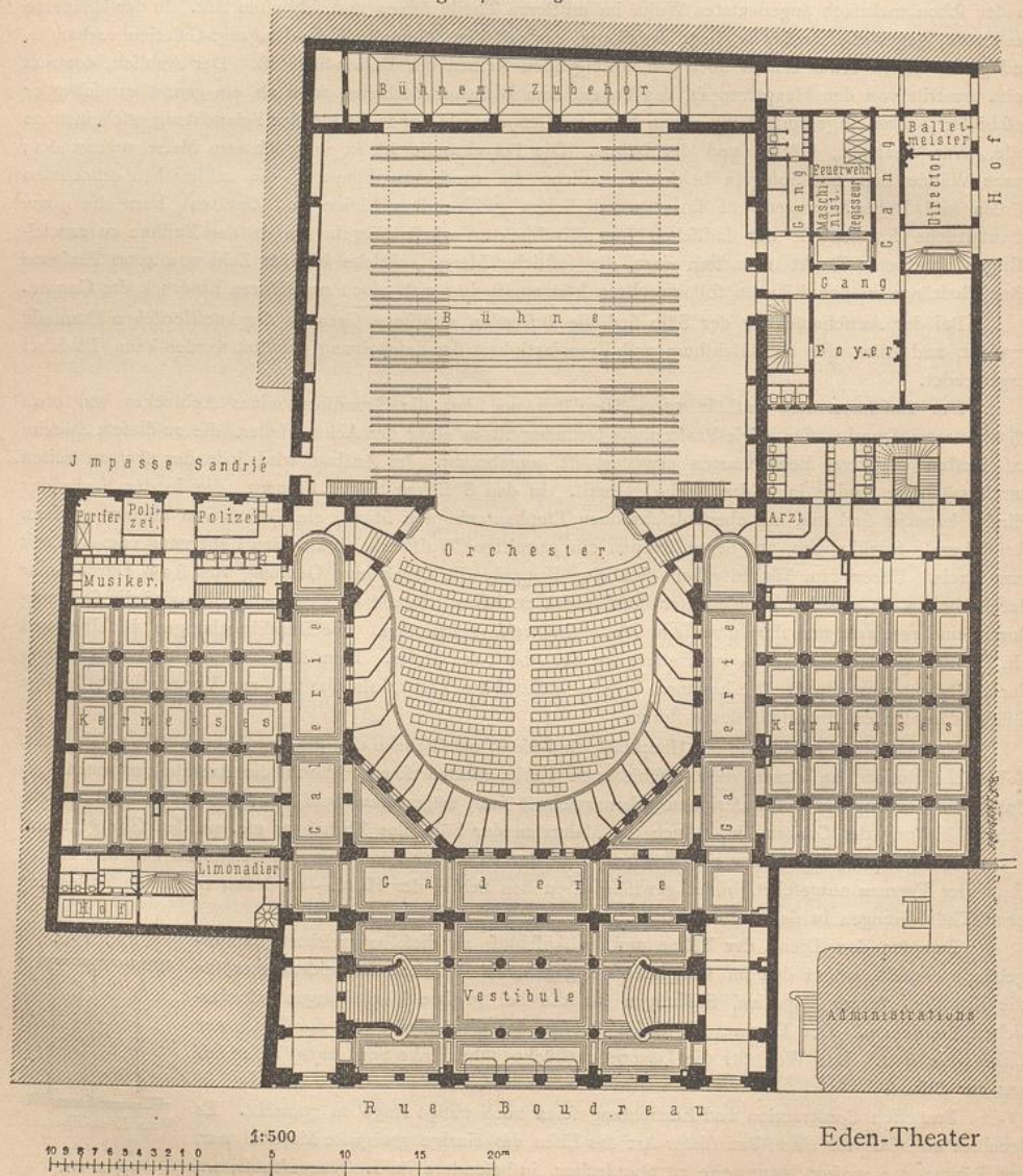
Fig. 141. Erdgeschoss.
