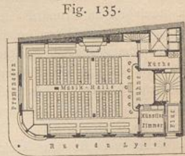
Fig. 135. Casino zu Troyes 115) . 1/500 n. Gr. Arch.: Fontaine.
