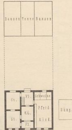
Westpreussisches Gehöft. (Brachlin — 5 ha.) ca. 1/1000 w. Gr.
