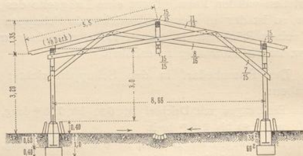
Dachbinder eines Karren- und Geräteschuppens. ca. \frac{1}{150} w. Gr. Arch.: Schubert.
