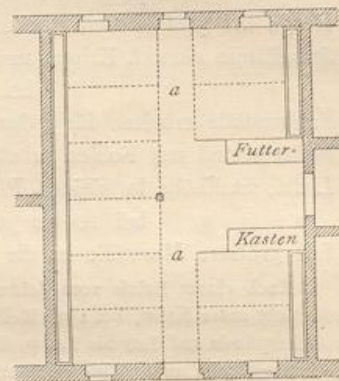
Querreihenstellung.
