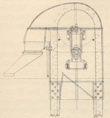
Elevator aus Dow's Getreidespeicher zu Brooklyn 60) . — \frac{1}{50} w. Gr.
