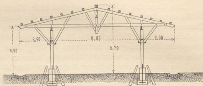
Dachbinder eines Karren- und Geräteschuppens. ca. \frac{1}{200} w. Gr.
