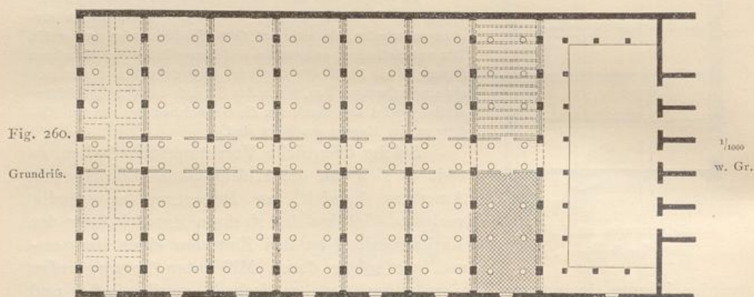
Unterirdisches Getreidemagazin zu Neapel 43) .
