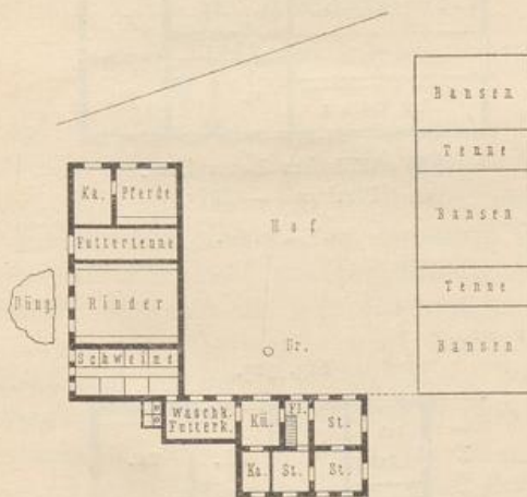
Lippisches Gehöft (Leiperode — 24 ha). ca. 1/100 w. Gr.
