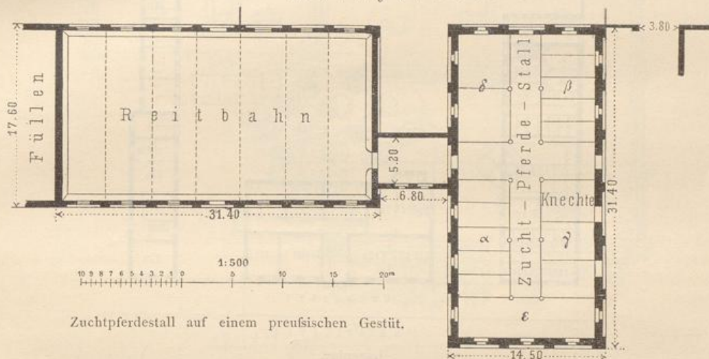
Fig. 73. Rossgarten.
