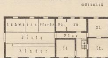
Westfälisches Bauernhaus. (Biechowo — 19 ha.) ca. 1/1000 w. Gr.
