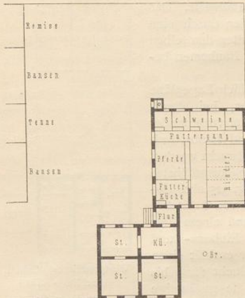
Westfälisches Gehöft (Bismarcksfelde — 15 ha). ca. 1/100 w. Gr.
