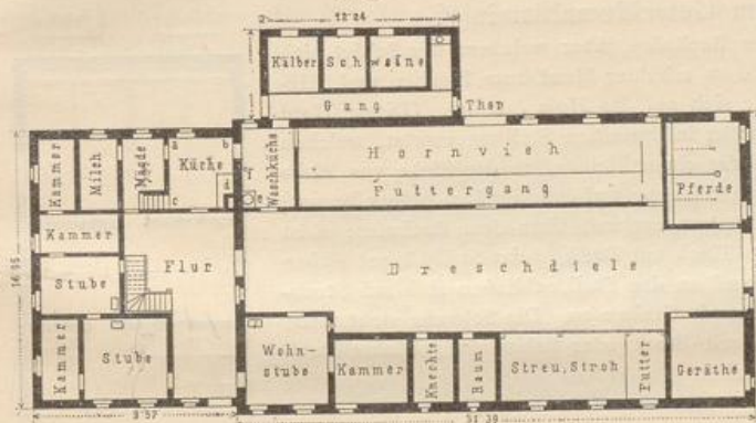
Ostfriesisches Platzgebäude. — 1/600 w. Gr.
