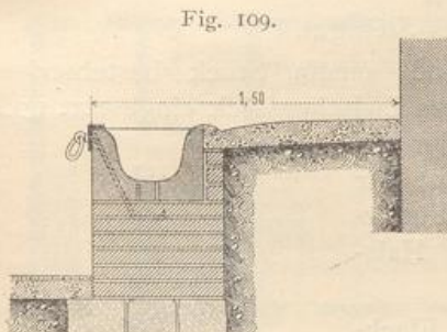
Krippe aus Ziegelformsteinen. 1/40 w. Gr.
