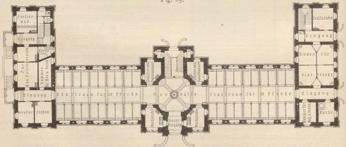
1:500 Herzogl. Marstallgebäude zu Gotha 26) .
