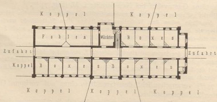
Zuchtpferdestall.
