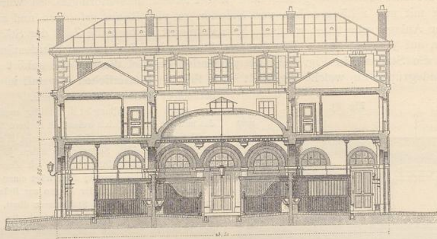
1:250 Stallung des vorm. Kaiserl. Marstalls zu Paris 21) . Arch.: Tétaz.
