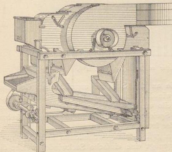
Staubfreie Aspirations-Reinigungs-Maschine (Separator) von Gebrüder Seck zu Dresden.
