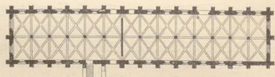
Getreidespeicher der Abtei zu Vauchlaire 30) . 1/1000 w. Gr.
