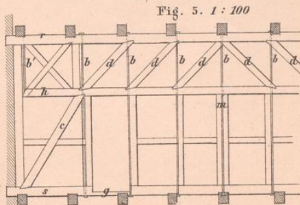
Fig. 5. 1:100
