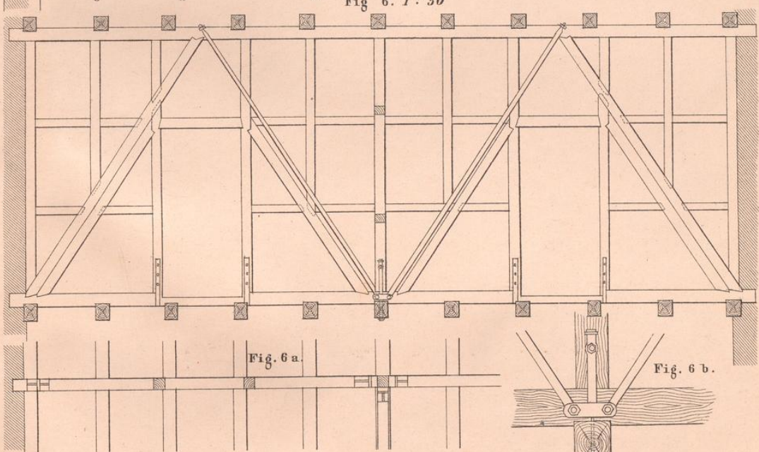
Fig. 6. 1:50
