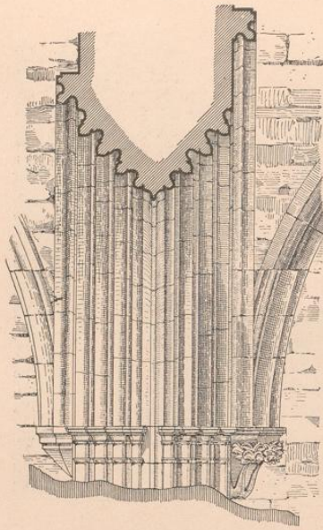
Abb. 65. Schnitt durch die Türe vom Kreuzgang nach dem Auslaß im Ostbau am Kreuzhof.
