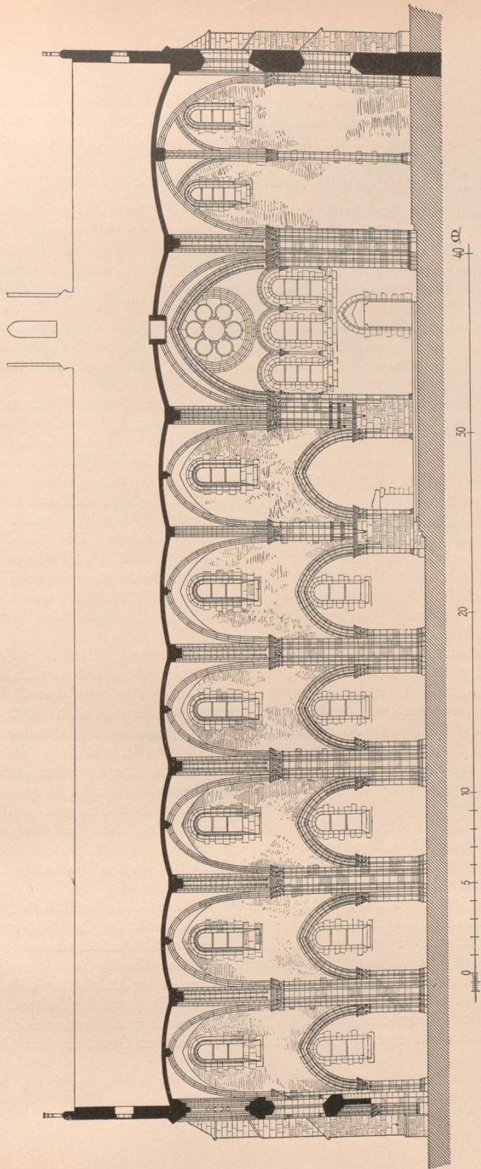
Abb. 96. Rekonstruktion der Kirche, Zustand um 1200, Längsschnitt A-B.
