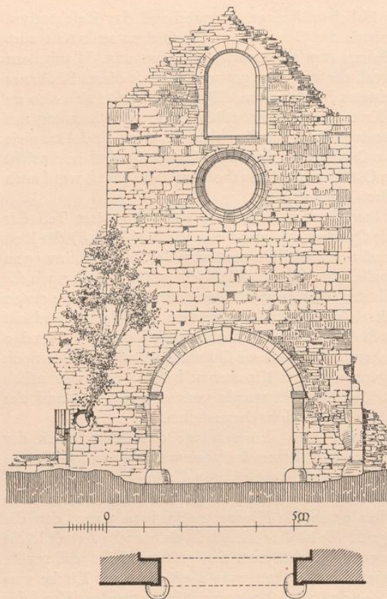
Abb. 91. Mittlerer Teil der Westwand des Ostbaus am Eingangshof, Ansicht und Grundriß.
