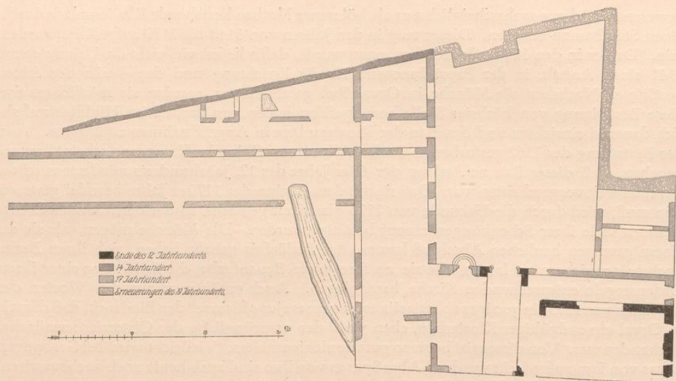
Abb. 90. Grundriß des Eingangshofs, jetziger Zustand.
