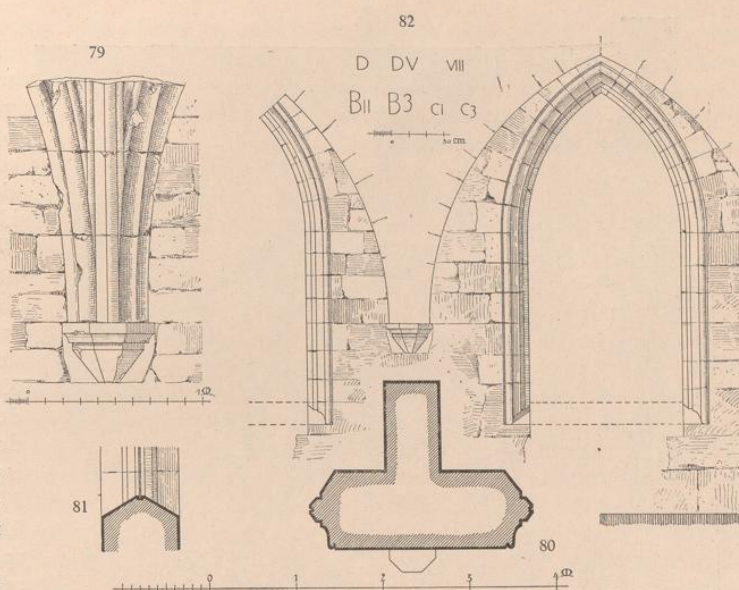
Abb. 79. Gewölbeanfang aus dem Kapitelsaal.
