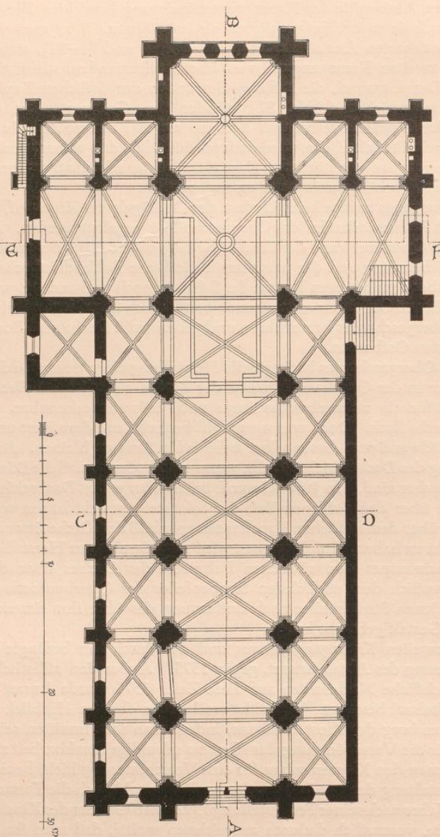
Abb. 94. Rekonstruktion der Kirche, Zustand um 1200, Grundriß.
