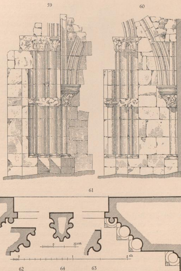
Abb. 59. Tür vom Kreuzgang zur Kirche, Schnitt. Abb. 60. Tür vom Kreuzgang zur Kirche, Ansicht. Abb. 61. Tür vom Kreuzgang zur Kirche, Grundriß. Abb. 62. Profil des Bogens über der Tür vom Kreuzgang zur Kirche. Abb. 63. Schildbogenprofil in den sieben östlichen Jochen des nördlichen Kreuzgangsflügels. Abb. 64. Rippenprofil in den sieben östlichen Jochen des nördlichen Kreuzgangsflügels.
