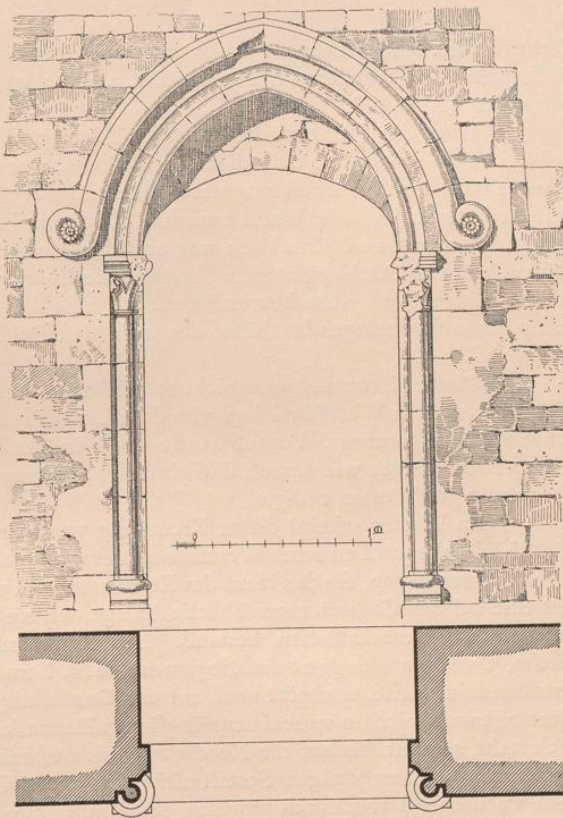
Abb. 89. Einzelheiten von einem Fenster des Empfangsgebäudes.
