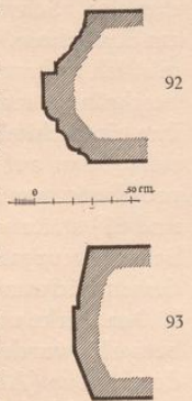
Abb. 92. Profil des Rundfensters in Abb. 91.
