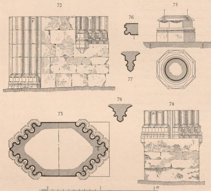
Abb. 72. Pfeiler zwischen der Mitteltür und dem südlichen Fenster in der Westwand des Kapitelsaals, Westansicht. Abb. 73. Pfeiler zwischen der Mitteltür und dem südlichen Fenster in der Westwand des Kapitelsaals, Grundriß. Abb. 74. Pfeiler zwischen der Mitteltür und dem südlichen Fenster in der Westwand des Kapitelsaals, Südansicht. Abb. 75. Mittelsäule im Kapitelsaal, Ansicht und Grundriß der Basis. Abb. 76. Schildbogen im Kapitelsaal. Abb. 77. Rippenprofil im Kapitelsaal und Auslaß. Abb. 78. Gurtbogenprofil im Kapitelsaal.
