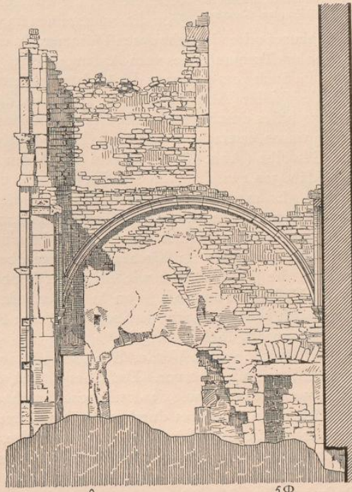
Abb. 84. Querschnitt durch den Ostsaal (Lesesaal) im Südbau am Kreuzhof, Blick nach Westen.
