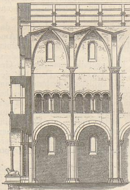
Inneres System des Domes von Parma. Längendurchschnitt. (Nach Osten.)
