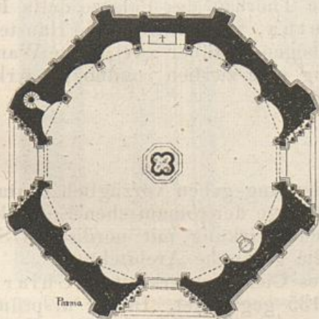
Grundriss des Baptisteriums von Parma. (Nach Osten.)
