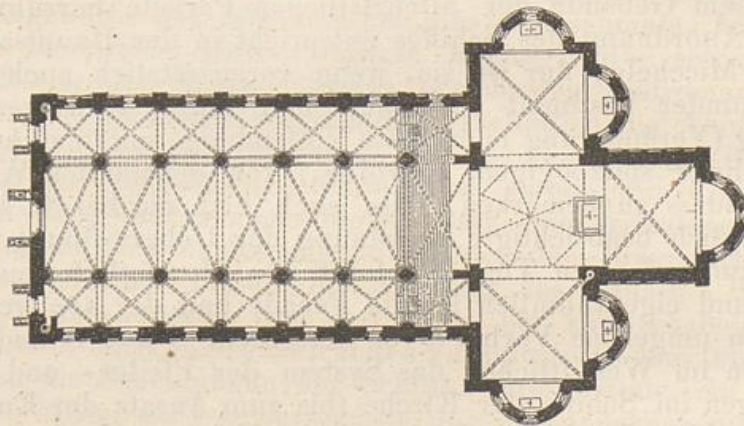
Grundriss des Domes von Parma. (Nach Osten.)
