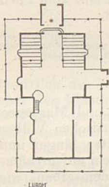
Grundriss der Kirche zu Lubom. (Nach Cuno.)
