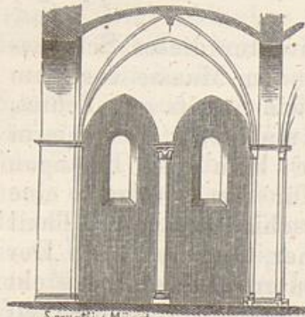
Servatius Münster. Servatiuskirche zu Münster. Inneres System des Schiffes. (Nach Lübke.)
