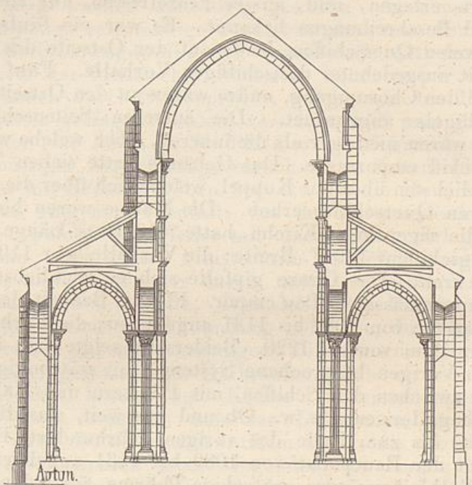
Querderschnitt der Kathedrale von Autun. (Nach Viollet-le-Duc.)
