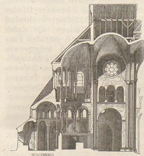
Kirche von Heisterbach. Durchschnitt des Chores. (Nach Boisserée.)
