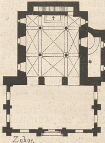
Grundriss der Kirche von Zabor. (Nach Woëel.)
